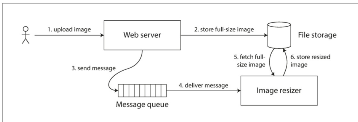
图9-5 Web服务器和图像调整器通过文件存储和消息队列进行通信，打开竞争条件的可能性。
