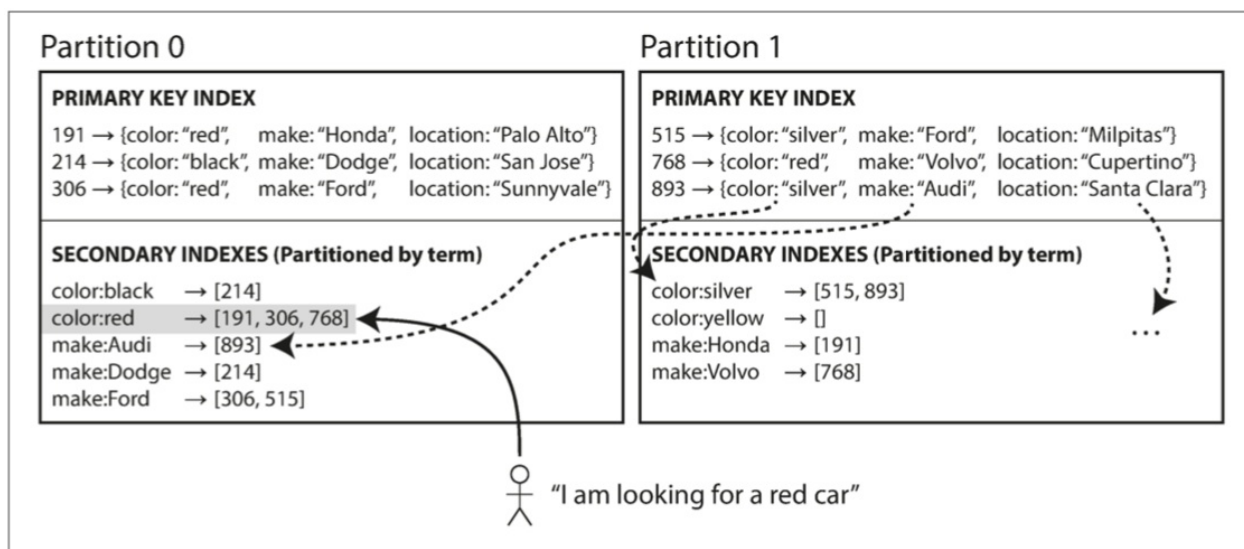
图6-5 按关键词对二级索引进行分区
